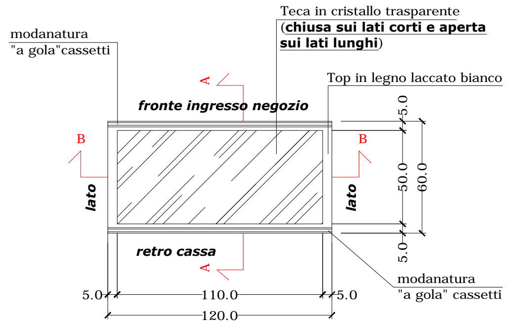
PIANTA
