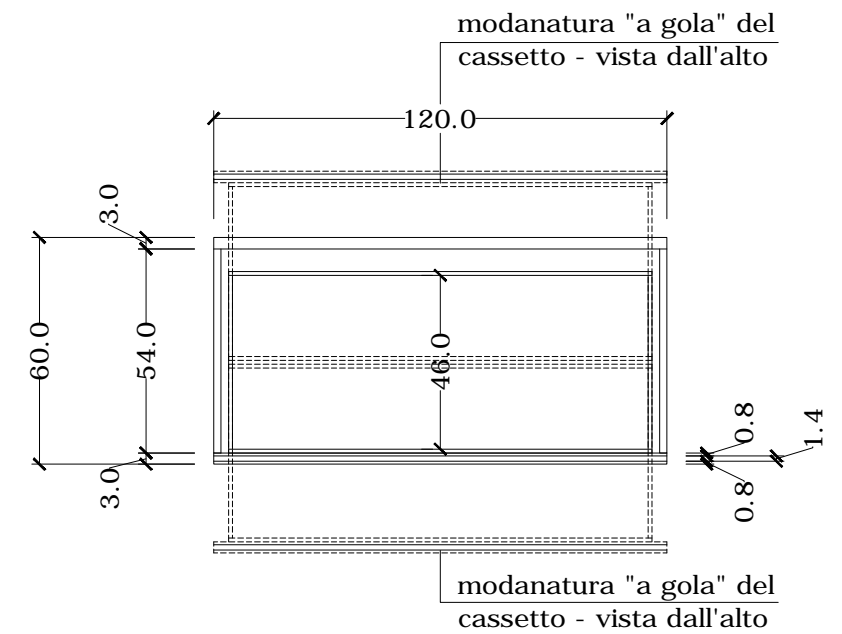
SEZIONE ORIZZONTALE
