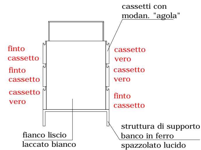
PROSPETTO LATERALE
